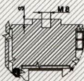
Insert type Detail A Scale: 1:1
