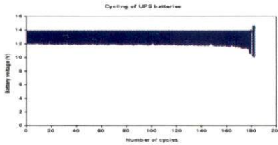
نمودار ولتاژ باتری در دوام چرخه ای
