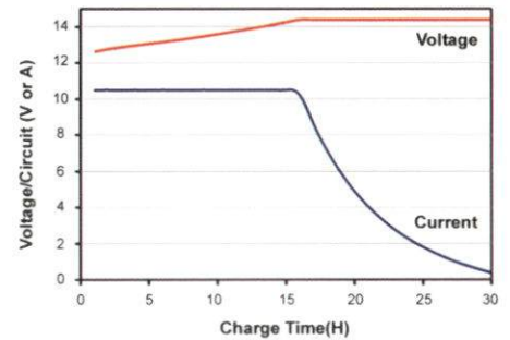
نمودارهای ولتاژ و جریان شارژ مجدد با مقادیر محدود شده
