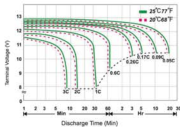
نمودار دشارژ
