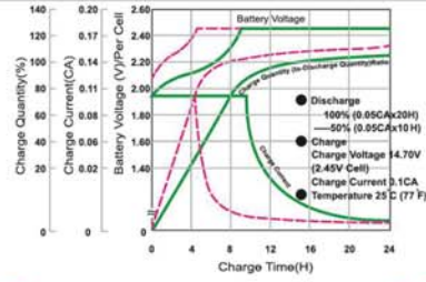
نمودار منحنی شارژ در حالت استفاده
