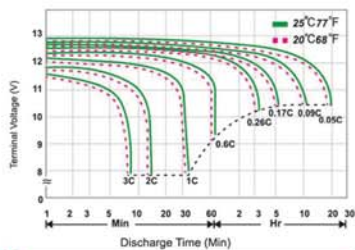
نمودار دشارژ
