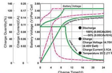
نمودار منحنی شارژ در حالت استفاده
