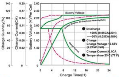
نمودار منحنی شارژ در حالت آماده بکار
