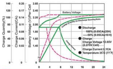
نمودار منحنی شارژ در حالت آماده بکار
